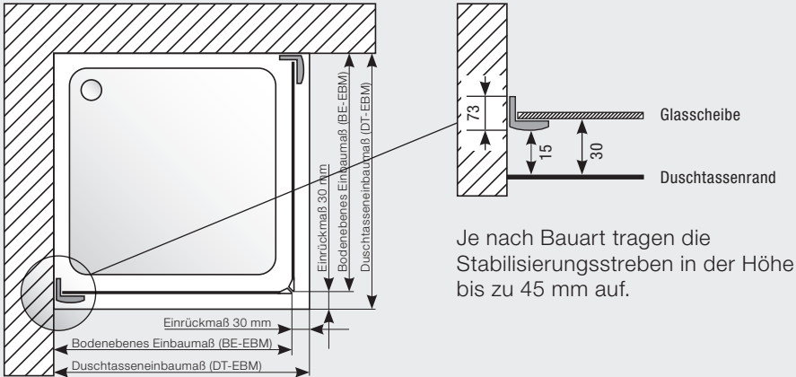
Montage auf Duschtasse
