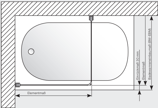
Montage auf Badewannenrand
