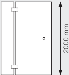
Festteil mit Drehtür (Bänderlösung)
