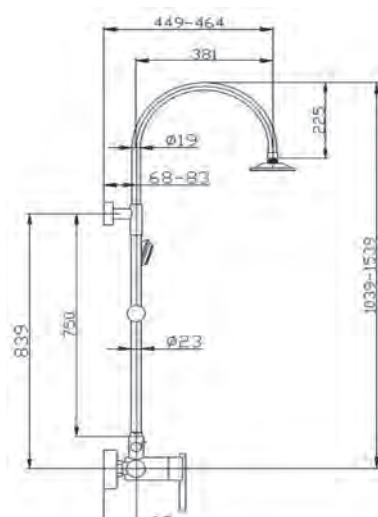
mit Einhebelmischer
