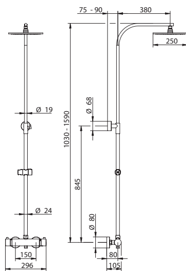
mit Thermostat
