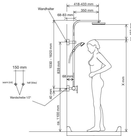
mit Einhebelmischer
